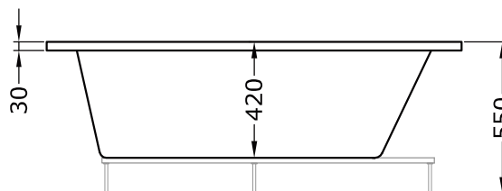
Alzado
