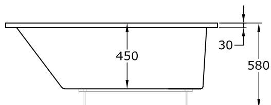
Alzado
