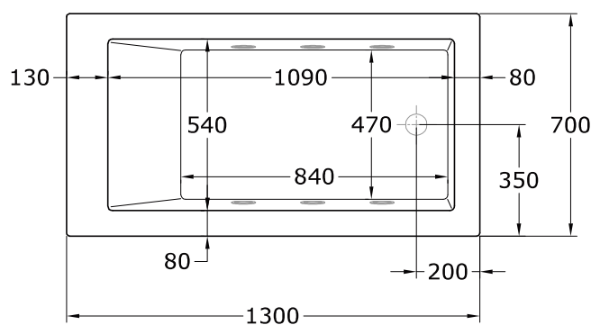
Planta
