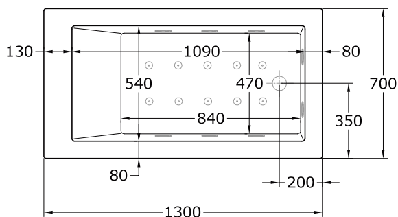
Planta
