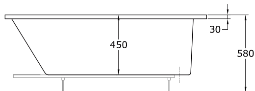
Alzado
