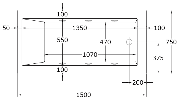
Planta
