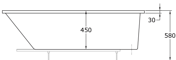
Alzado
