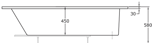
Alzado
