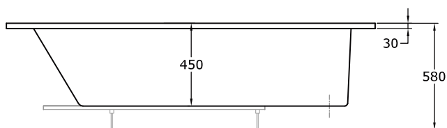
Alzado
