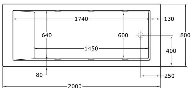
Planta
