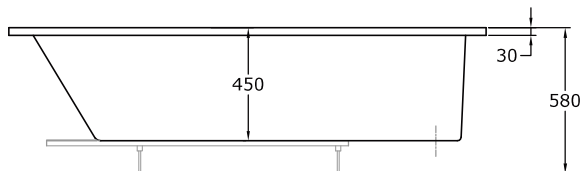
Alzado
