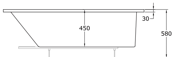
Alzado
