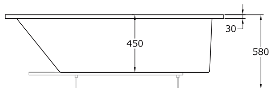
Alzado
