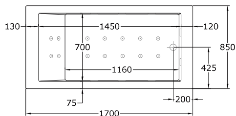
Planta
