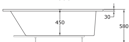
Alzado
