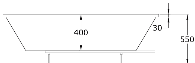
Alzado
