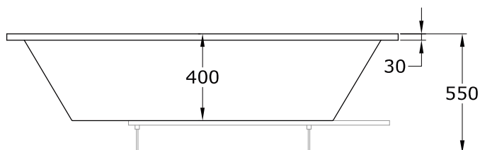
Alzado
