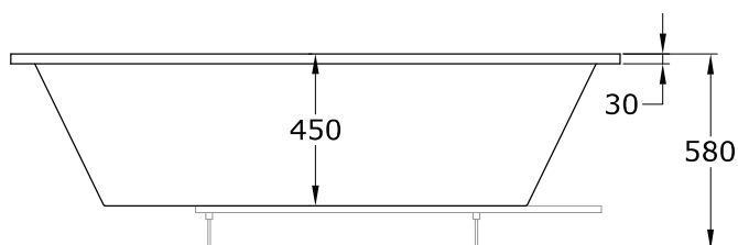
Alzado
