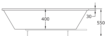
Alzado
