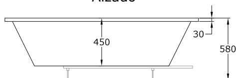
Alzado
