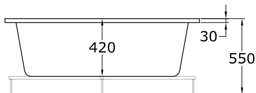
Alzado
