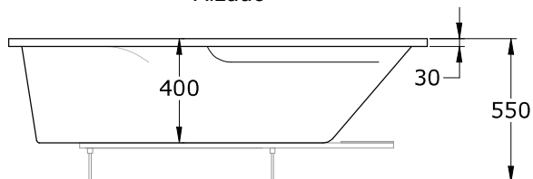
Alzado
