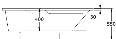
Alzado
