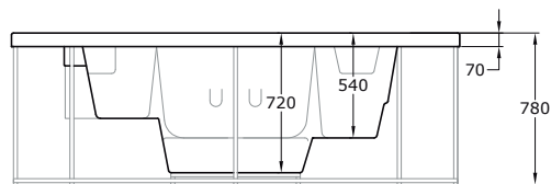
Alzado
