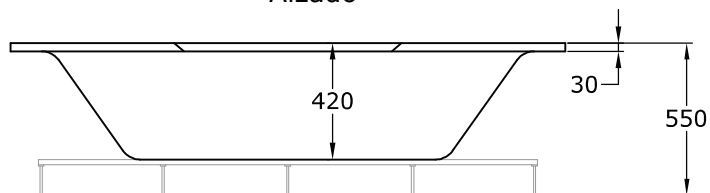
Alzado
