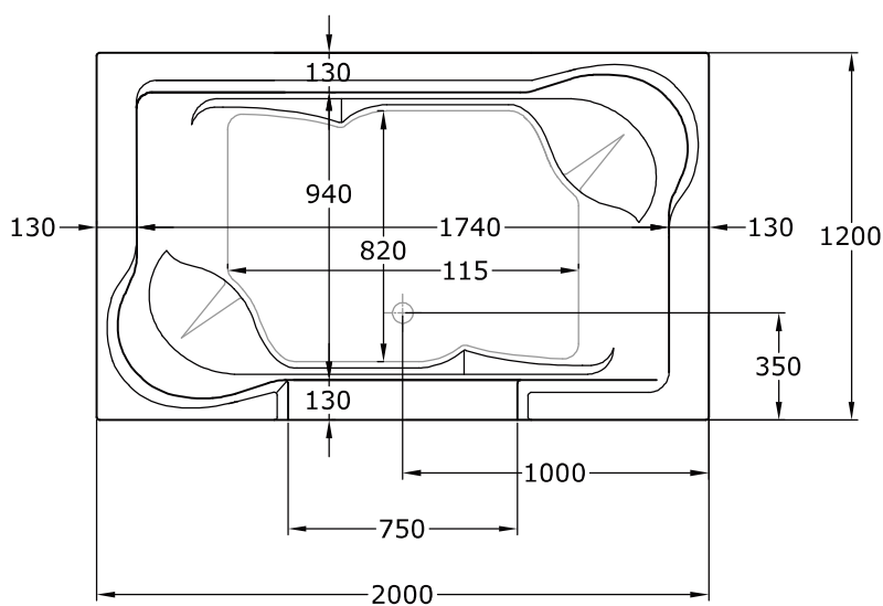
Planta
