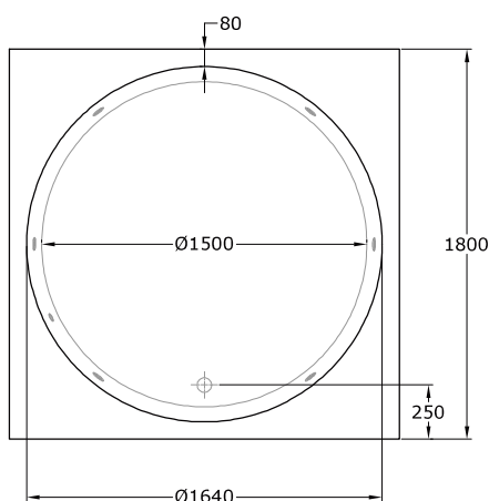
Planta
