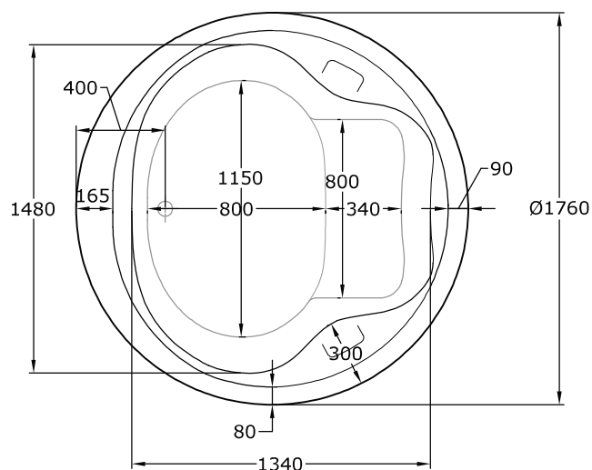
Planta
