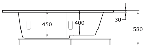
Alzado
