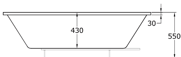
Alzado
