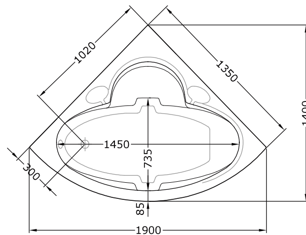
Planta
