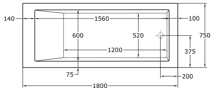
Planta
