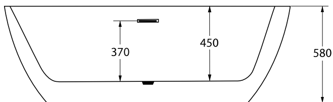
Sección
