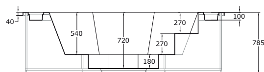
Sección
