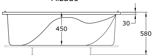
Alzado
