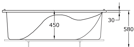
Alzado
