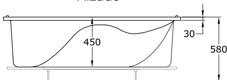
Alzado
