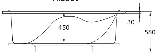
Alzado
