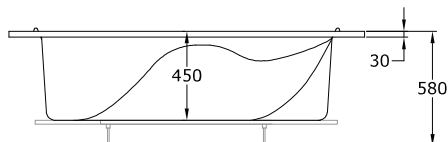
Alzado
