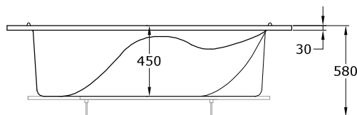
Alzado
