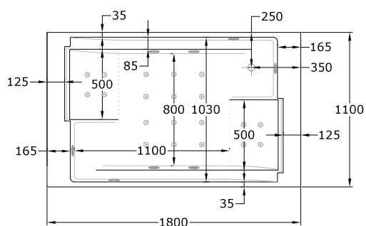
Planta
