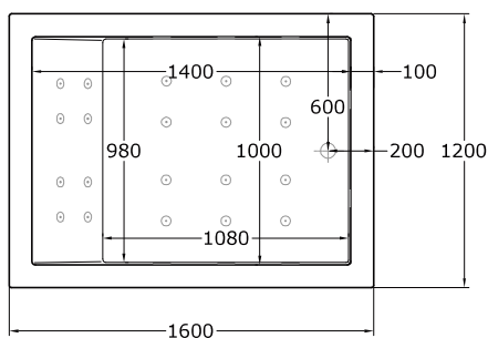
Planta
