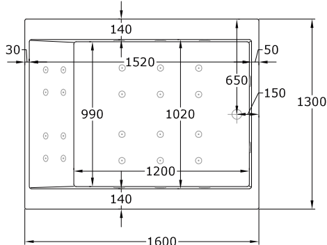
Planta
