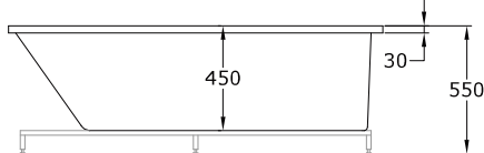
Alzado - Sección
