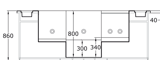
Sección
