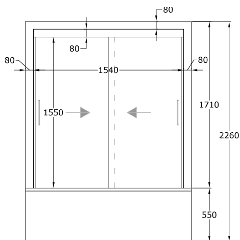
Alzado
