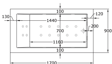
Planta bañera
