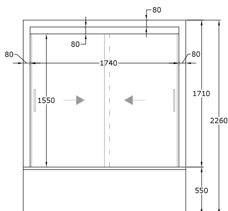
Alzado
