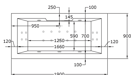
Planta bañera
