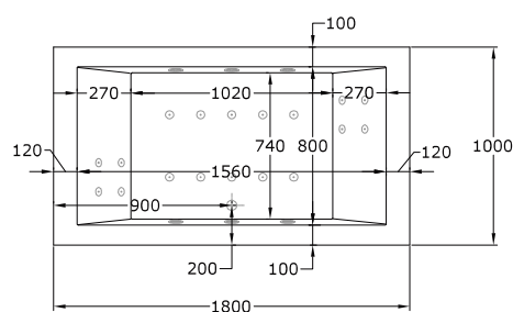
Planta bañera
