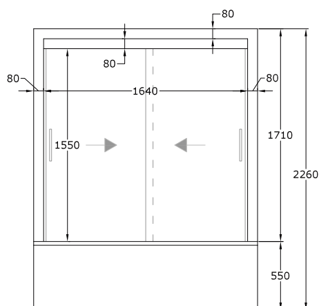
Alzado
